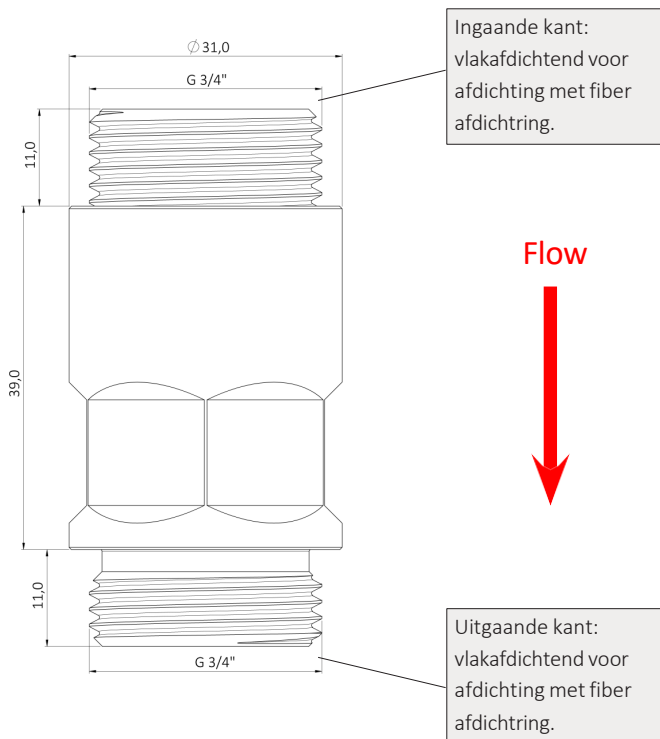
Afbeelding: Control Flow Inline 1P 3/4" (afmetingen in mm)
