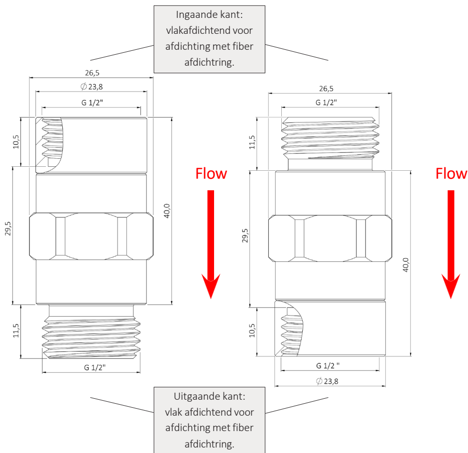
Afbeelding: Control Flow Inline 1P 1/2" f-m (afmetingen in mm)
